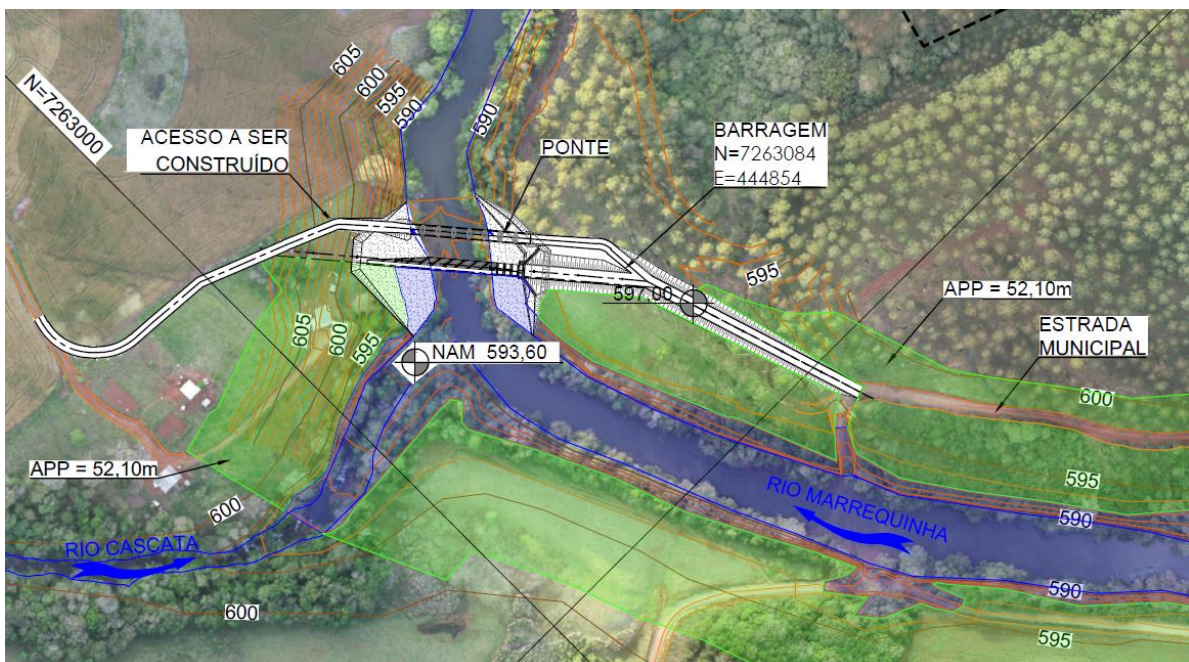
Figura 32: Ponte a ser construída à jusante do barramento da CGH Santa Jacinta.
