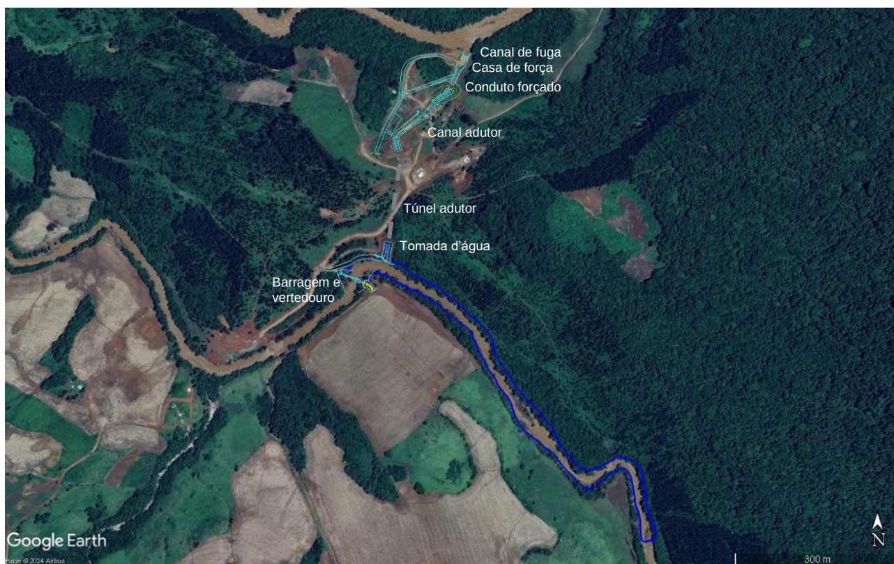
Figura 4: Arranjo geral e alagamento da CGH Santa Jacinta.
