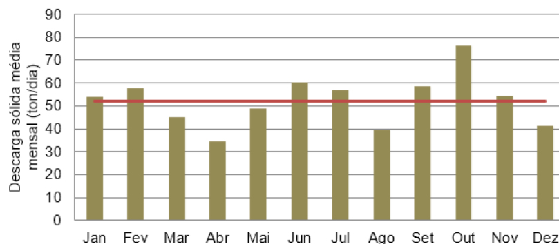
Figura 43: Descarga sólida calculada para a CGH Santa Jacinta.
